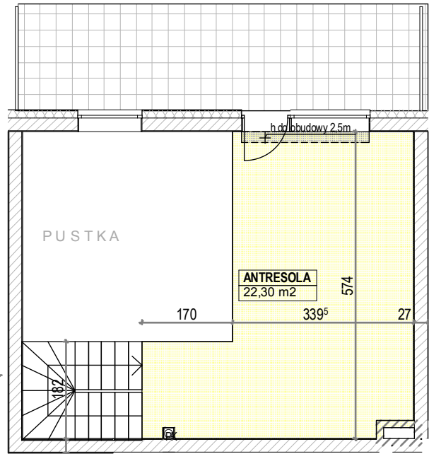
RZUTY MIESZKANIA
