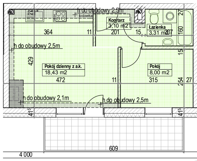
RZUT MIESZKANIA
