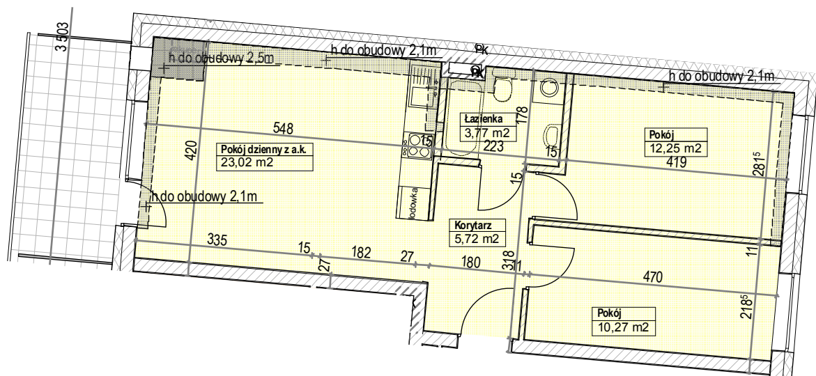
RZUT MIESZKANIA
