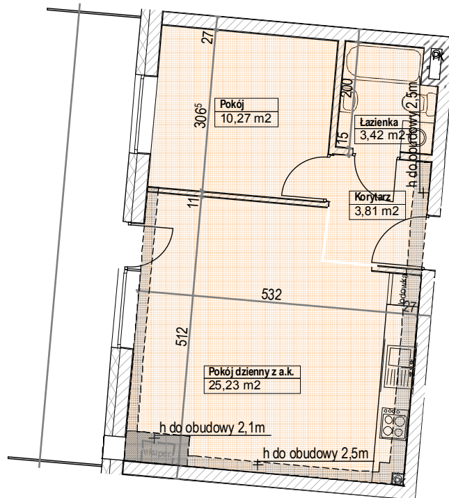
RZUT MIESZKANIA
